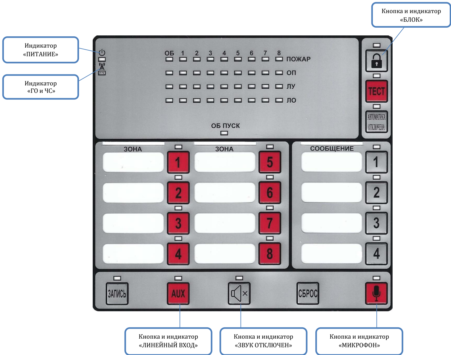
Рисунок 1. Органы управления и индикации блока управления
