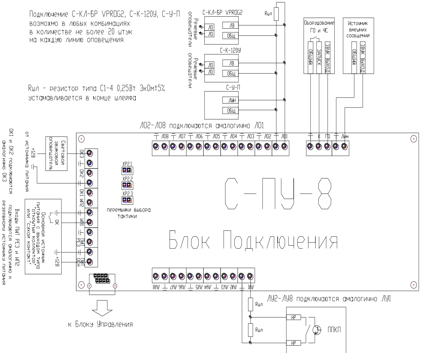
Рисунок 5. Схема подключений прибора С-ПУ-8
